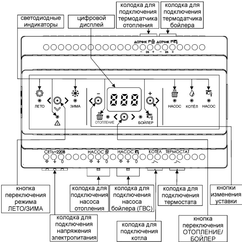
Рисунок 1 — Общий вид передней панели изделия
