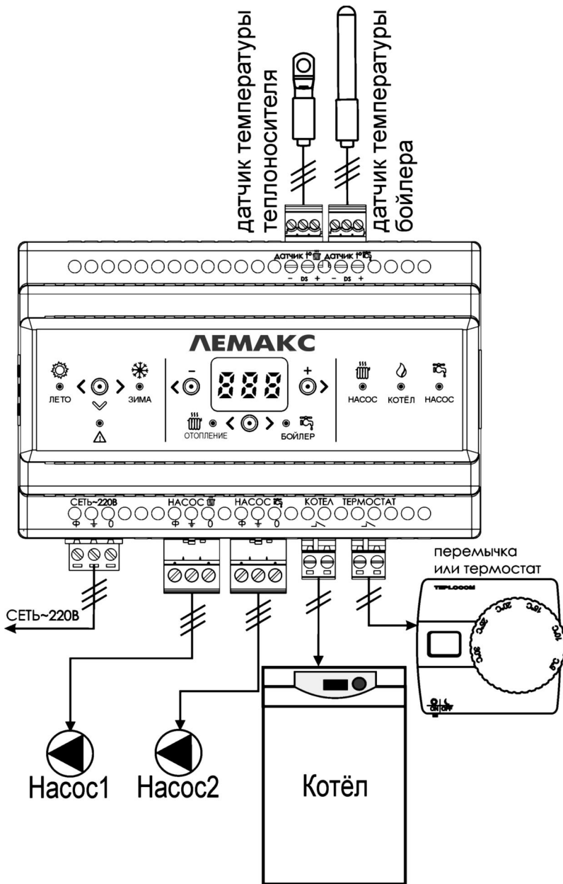
Рисунок 4 - Схема подключения
